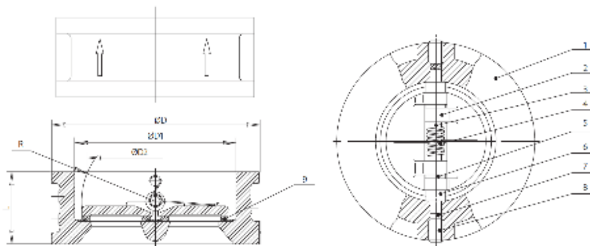
Рисунок 1. Конструкция клапана
